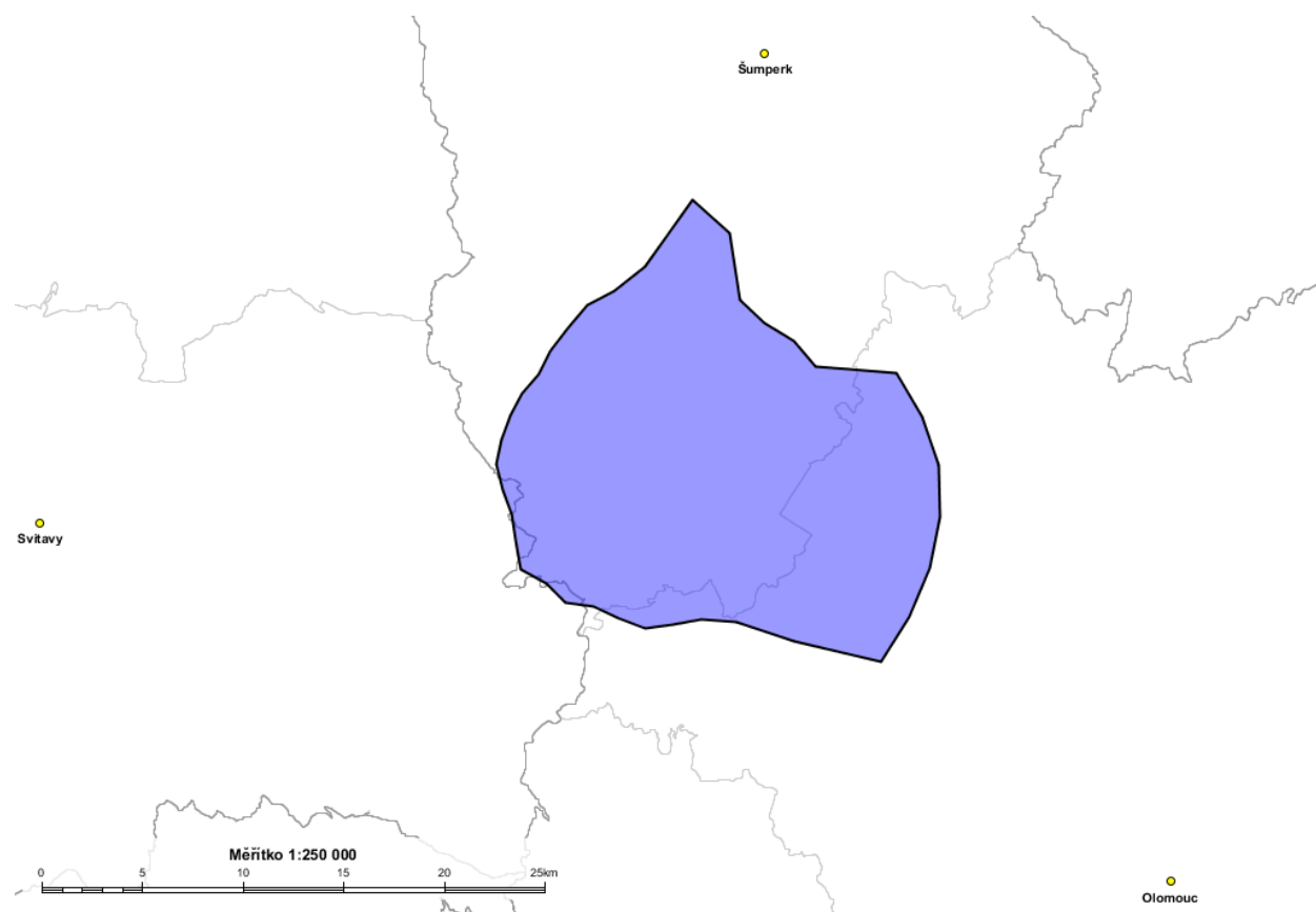
Příloha č. 11 (předpokládaný územní rozsah vysílače Mohelnice 2 97,8 MHz / 400 W)
