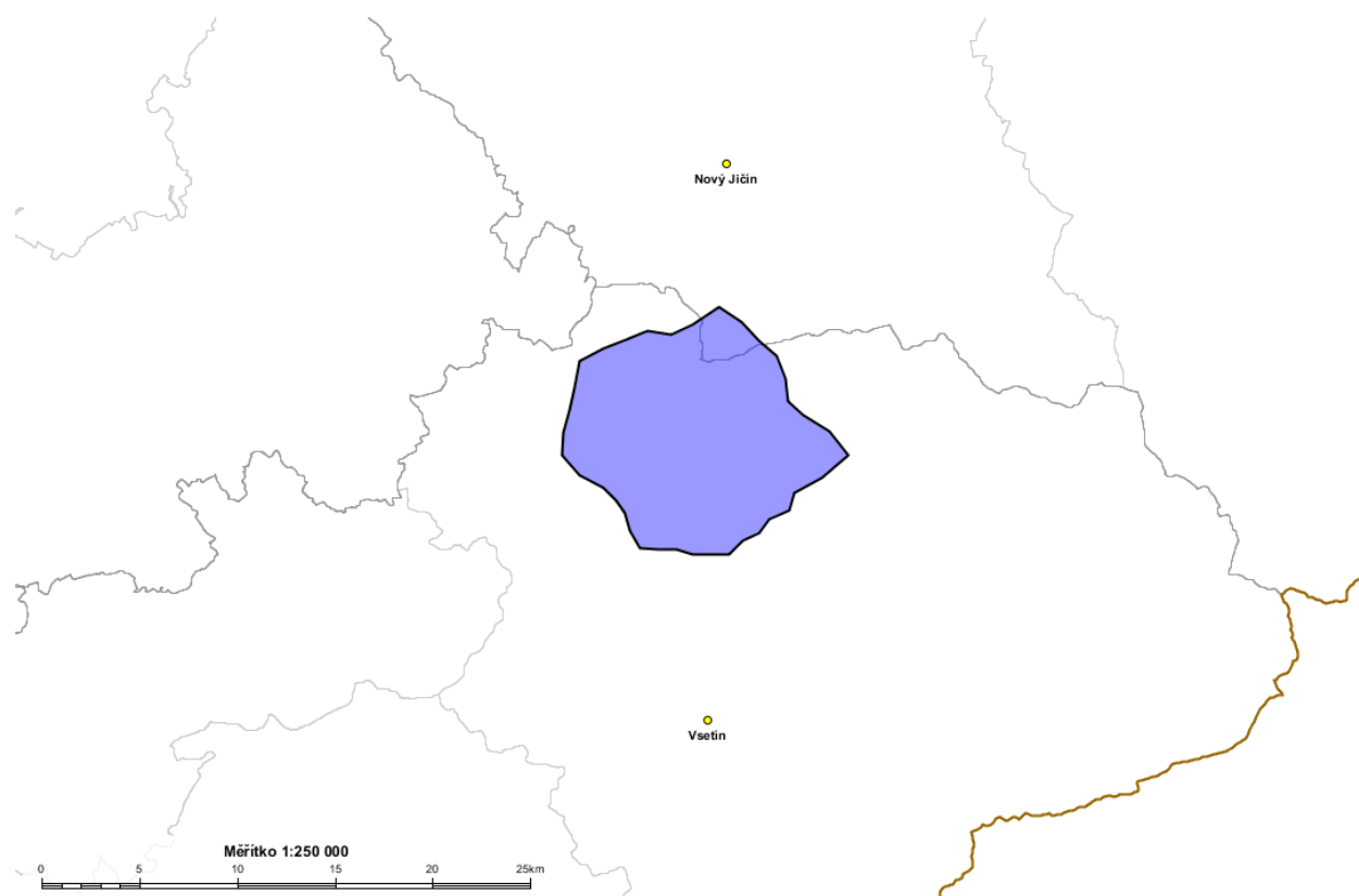
Příloha č. 19 (předpokládaný územní rozsah vysílače Valašské Meziříčí Štěpánov 93,5 MHz / 100 W)
