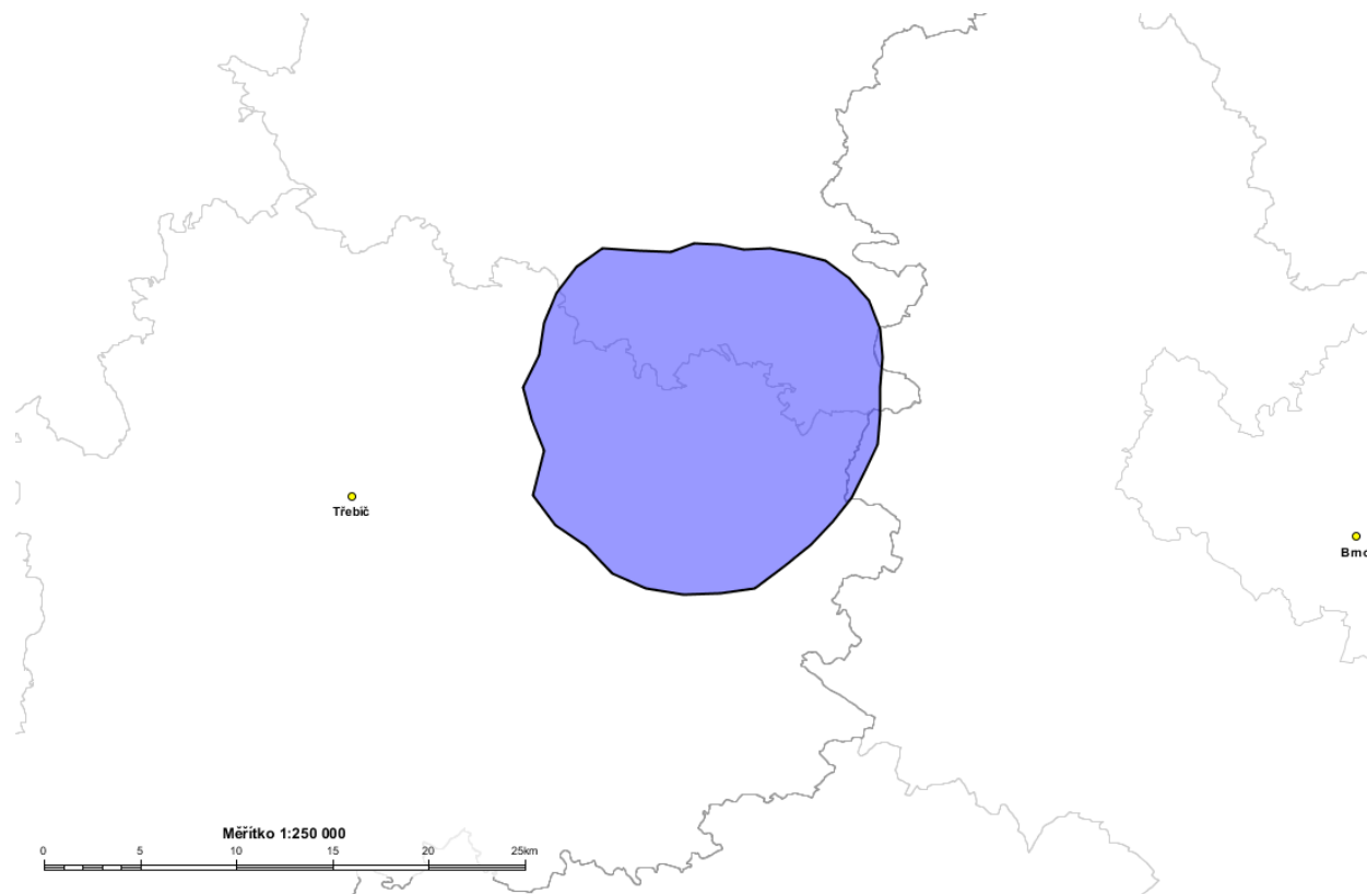
Příloha č. 21 (předpokládaný územní rozsah vysílače Velká Bíteš Číkov 93,7 MHz / 100 W)
